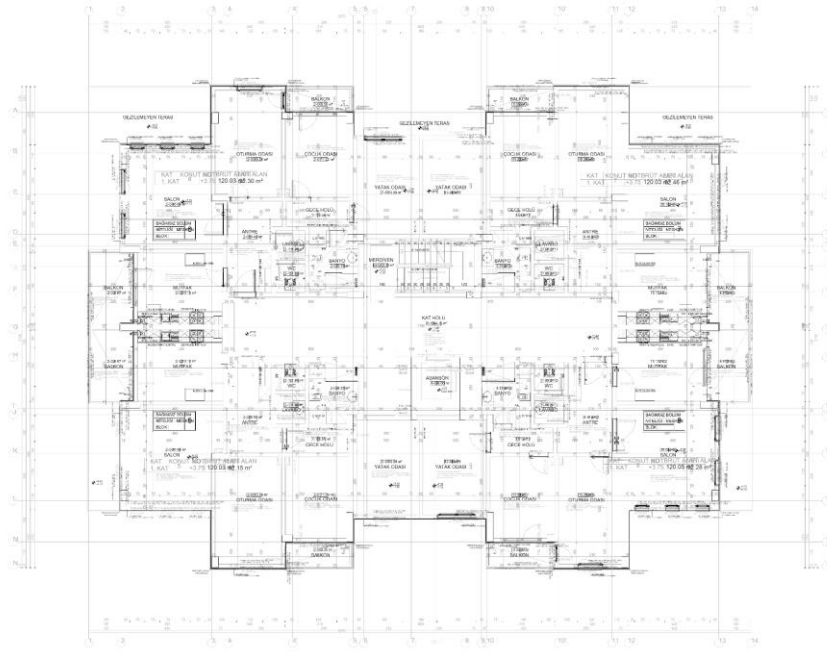
İKİNCİ KAT PLANI Ölçek:1/50 D BLOK
